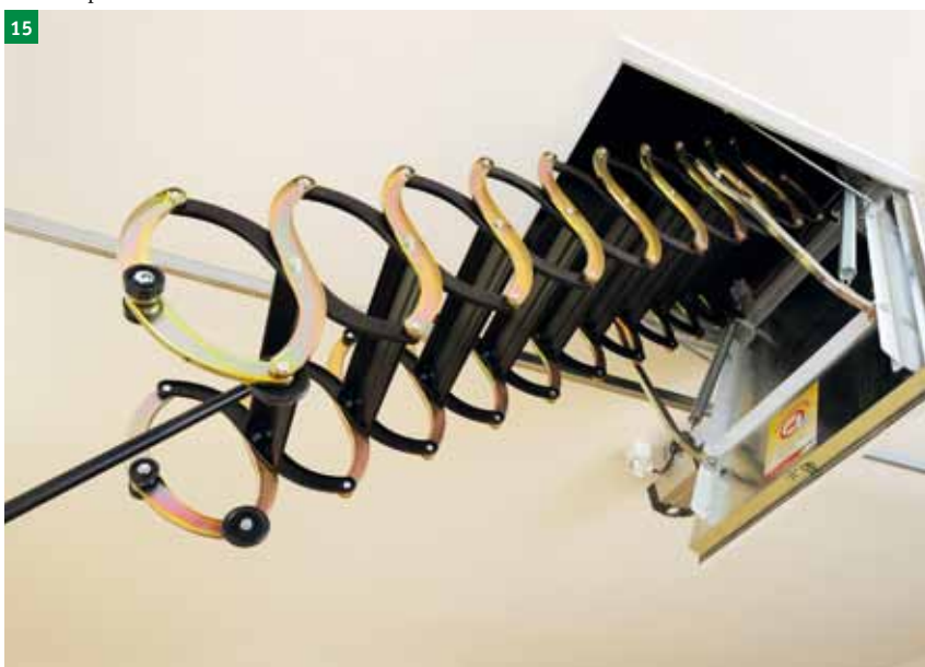
15 S pomočjo palice potisnite stopnice navzgor
