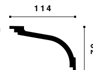
Z17 ARSTYL® 79 x 114 x 2000 mm
