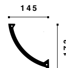
L3 ARSTYL® 173 x 145 x 2000 mm
