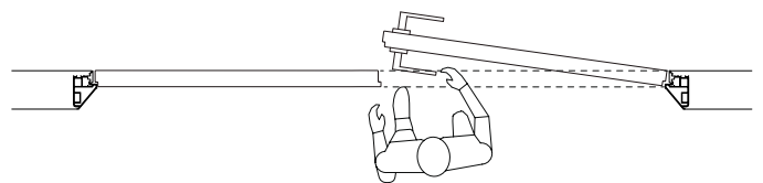
RIGHT PUSH DOOR - LEFT DOOR FIXED
